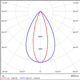
Calumma L SC RGBW 6500K 30x30dg
