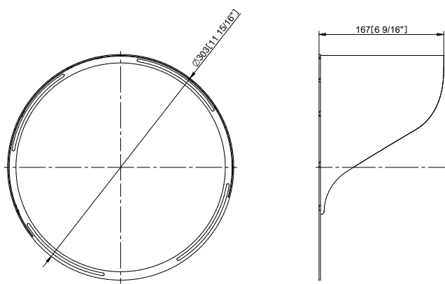
Half Top Hat
