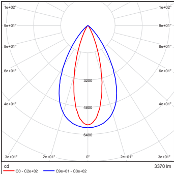
Calumma L MC RGBW 6500K 30x30dg
