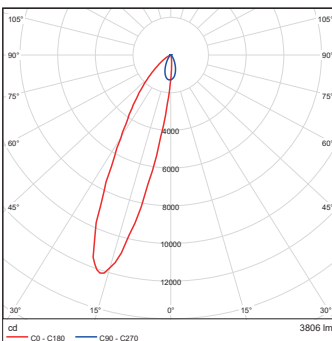
Eminere Side 4 RGBCW WallWasher
