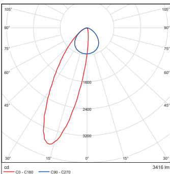
Eminere Side 4 RGBCW Wide WallWasher
