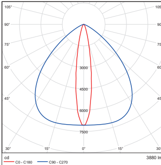
Eminere Side 4 RGBCW 15dg x 90dg
