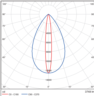
Eminere Side 4 RGBCW 10dg x 60 dg
