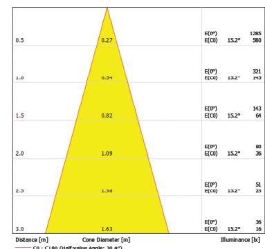
ArcLink 3 RGB - Non Optic
