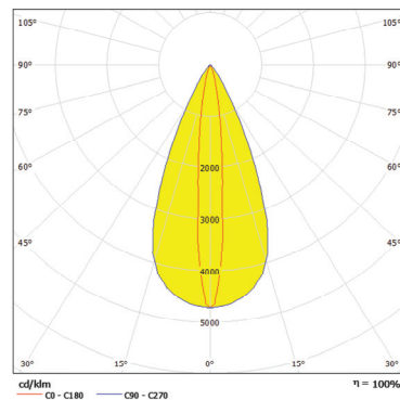
ArcLink 3 RGB - 46°x11°
